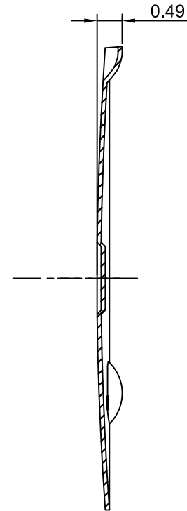
SECTION A-A
