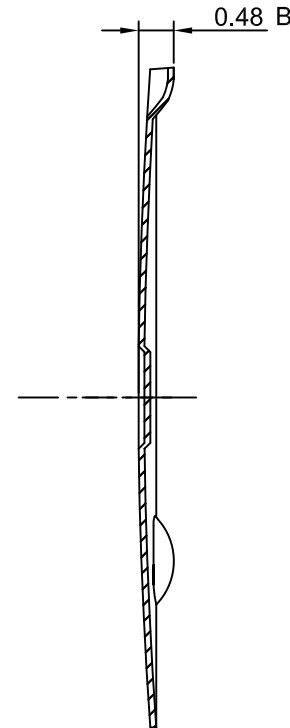
SECTION A-A
