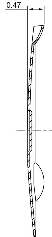
SECTION A-A
