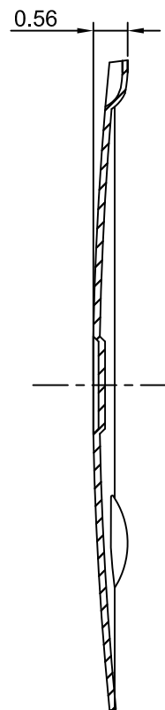
SECTION A-A
