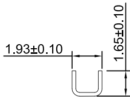
A-A SECTION
