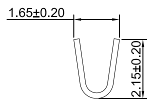
A-A SECTION
