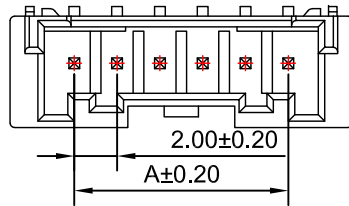
2PIN~6PIN
