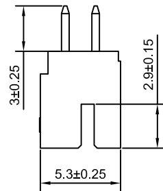
2PIN
