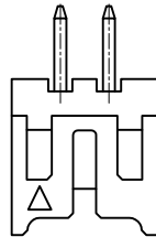
2PIN
