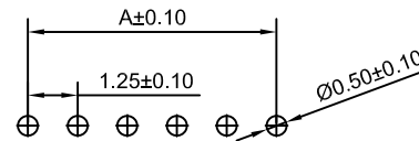
P.C.B LAYOUT
